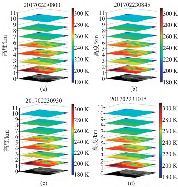
Fig. 4 Temperature profiles at different heights and times 图4 不同时间高度温度反演分布图
