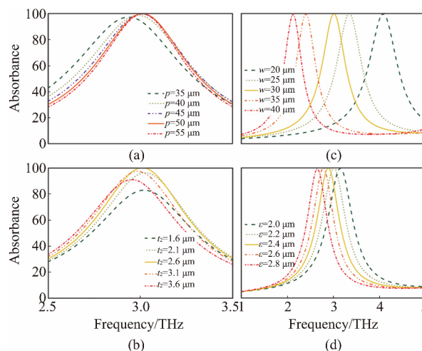
图 2 数值仿真得到的不同结构几何参数和介质层材料的吸收光谱。(a) 金属条 w = 30 \mu\text{m} , 介质层厚度 t_2 = 2.6 \mu\text{m} , 介电常数 \varepsilon = 2.2 , 改变金属条状结构的周期 p = 35\text{--}55 \mu\text{m} ; (b) 金属条状结构周期 p = 50 \mu\text{m} , 金属条 w = 30 \mu\text{m} , 介电常数 \varepsilon = 2.2 , 改变介质层的厚度 t_2 = 1.6\text{--}3.6 \mu\text{m} ; (c) 金属条状结构周期 p = 50 \mu\text{m} , 介质层厚度 t_2 = 2.6 \mu\text{m} , 介电常数 \varepsilon = 2.2 , 改变金属条的宽度 w = 20\text{--}40 \mu\text{m} ; (d) 金属条状结构周期 p = 50 \mu\text{m} , 金属条 w = 30 \mu\text{m} , 介质层厚度 t_2 = 2.6 \mu\text{m} , 改变介质层材料的介电常数 \varepsilon = 2.0\text{--}2.8
