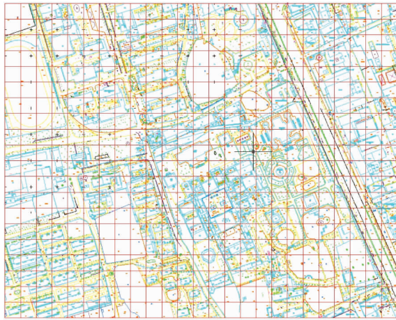
图1 研究区 30 m x 30 m 格网划分示意图 Fig. 1 Schematic diagram of a 30 m x 30 m grid division
