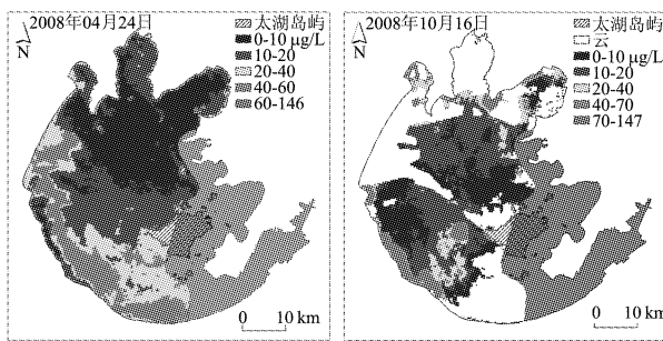
图4 基于 MERIS 遥感影像的 2008 年 04 月 24 日和 10 月 16 日的叶绿素 a 浓度空间分布 Fig. 4 Spatial distribution of chlorophyll a concentration using MERIS images on 24 April and 16 October 2008
