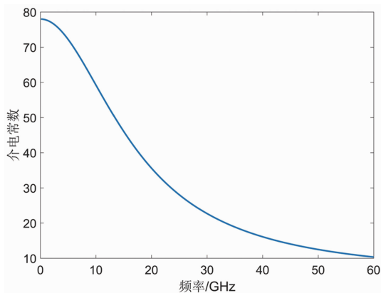
图 4 水的介电常数随频率的变化曲线
