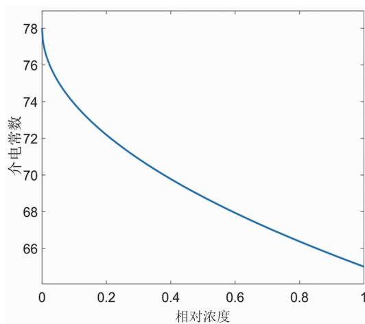
图 6 乳糖溶液的介电常数随浓度的变化曲线
