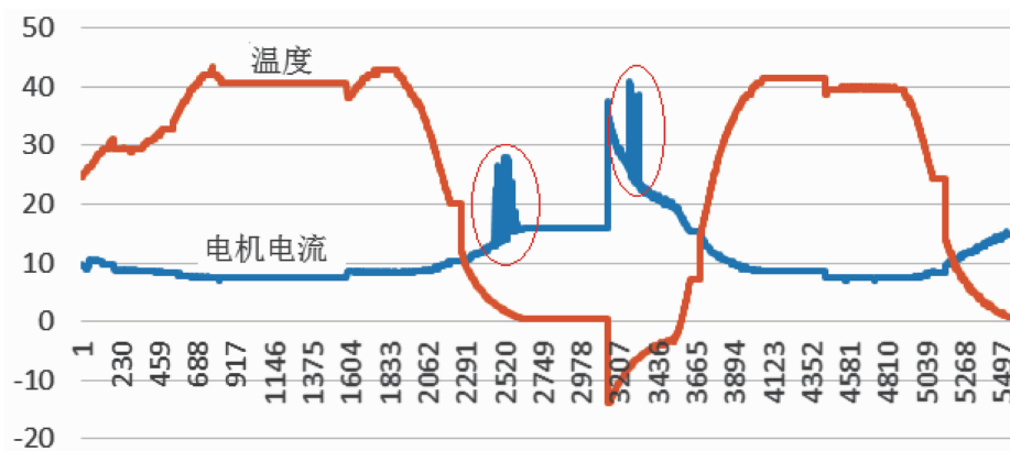
图 2 热真空试验中的红外地平仪电机电流遥测波动曲线(mA-℃)
