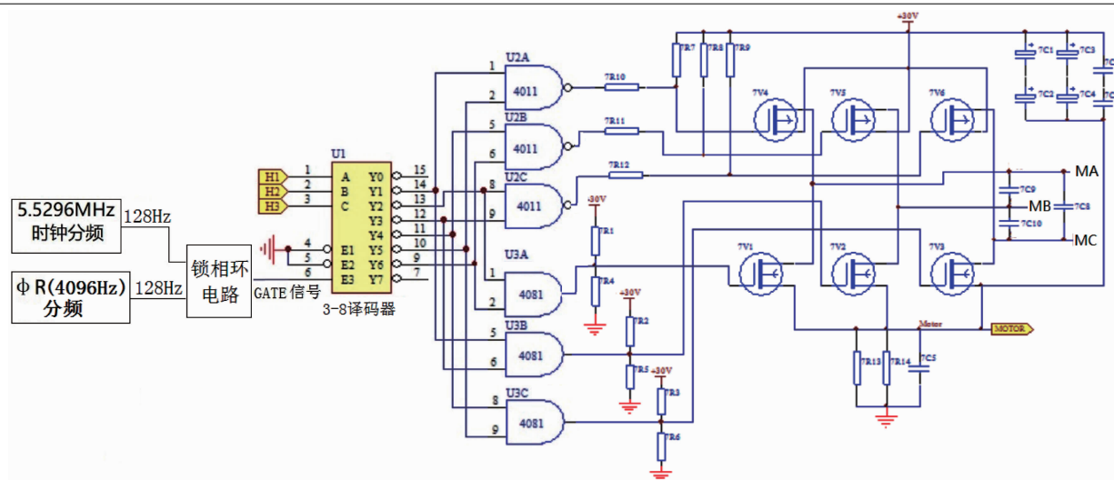
图 3 红外地平仪电机驱动和稳速电路的原理图
