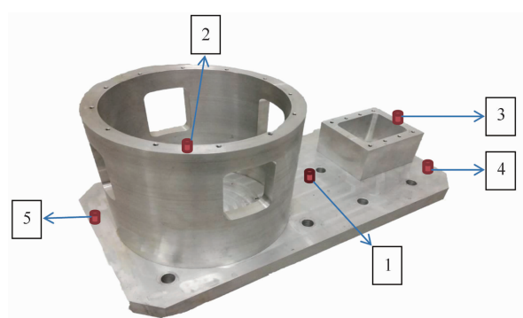
图 2 工装夹具图
