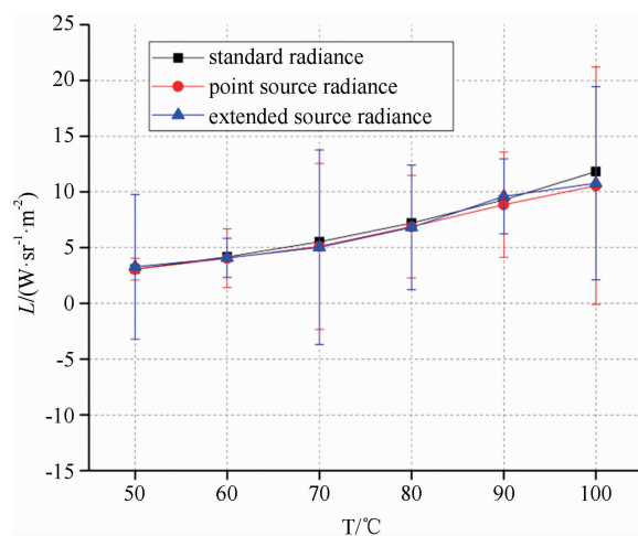
图 10 在积分时间为 3000\ \mu\text{s} 时两种目标的辐射测量比对结果
