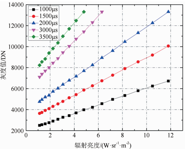
图 5 辐射定标结果
