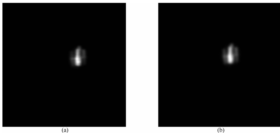
图 2 长波红外成像仪对哈勃空间望远镜的成像效果: (a)探测波段为 8.35~9.13 \mu\text{m} ; (b)探测波段为 11.1~12.2 \mu\text{m}
