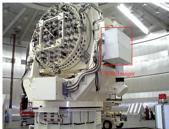
图 1 毛伊岛观测站的 3.67 m 长波红外成像仪
