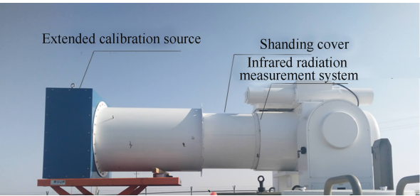
图 4 辐射定标现场
