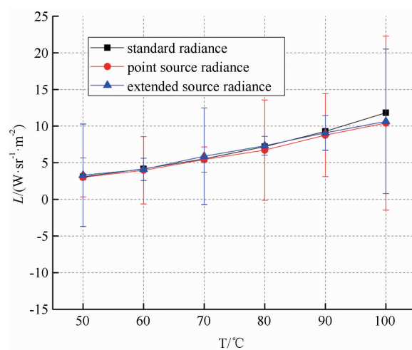
图 9 在积分时间为 2000\ \mu\text{s} 时两种目标的辐射测量比对结果
