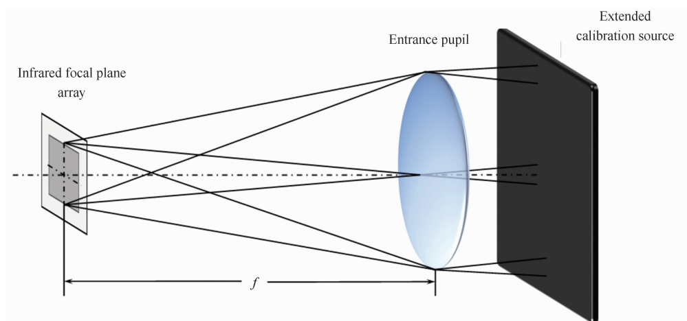
图 3 外置扩展源定标法的示意图
