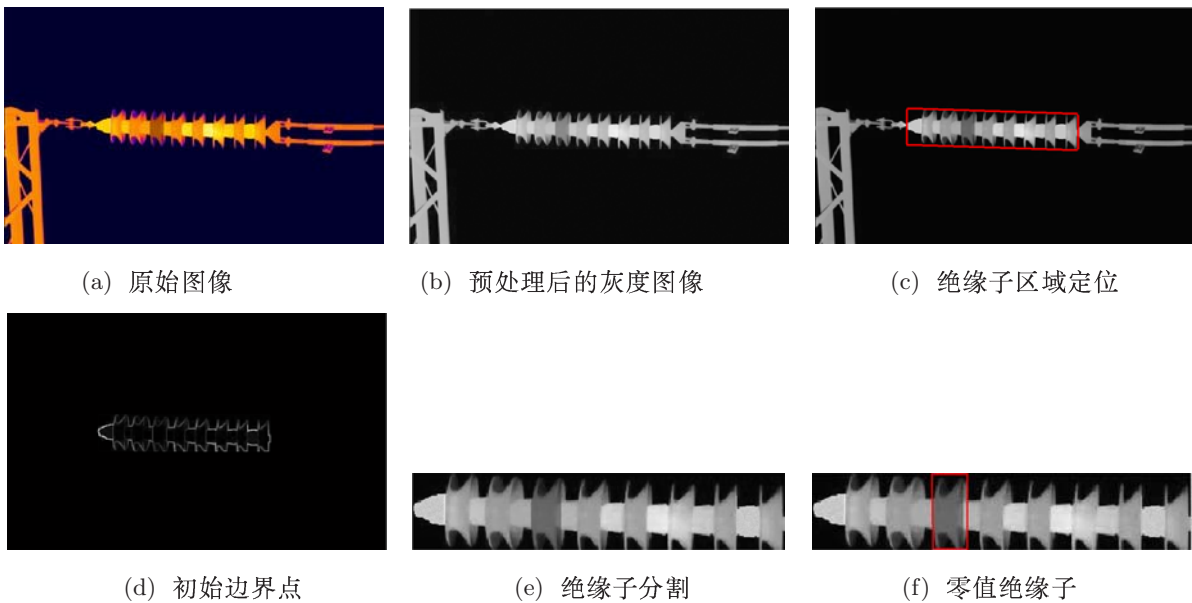
图 2 零值绝缘子的检测
